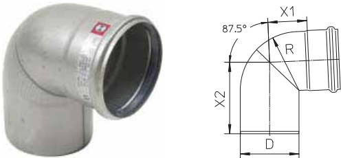
BEND 87.5° TYPE 820
