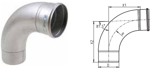
BEND MED STOR RADIUS 87.5° TYPE 820
