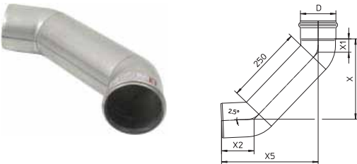
LANGBEND 87.5° TYPE 821
