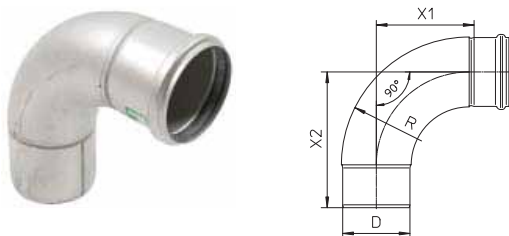
BEND MED STOR RADIUS 90° TYPE 825
