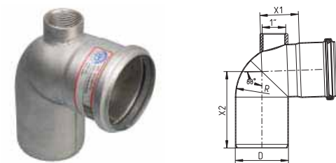
BEND 87.5° MED TILGANG TYPE 823
