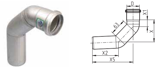
LANGBEND 87.5° TYPE 821
